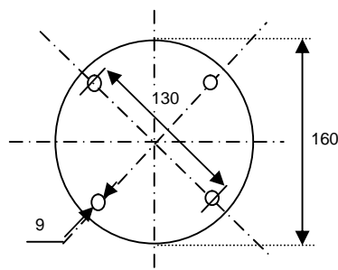
Dimensiones flange 71
