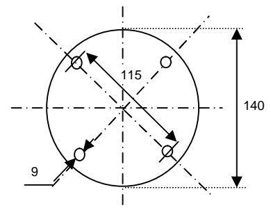
Dimensiones flange 63
