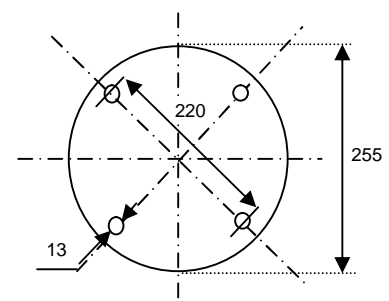
Dimensiones flange 250
