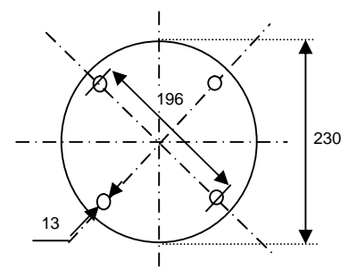
Dimensiones flange 230
